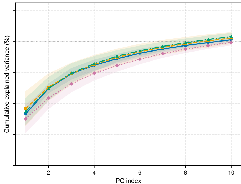
(B) PCA — pocket
